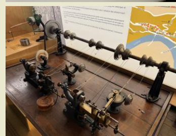
machine pour percer le diamant de la filière
